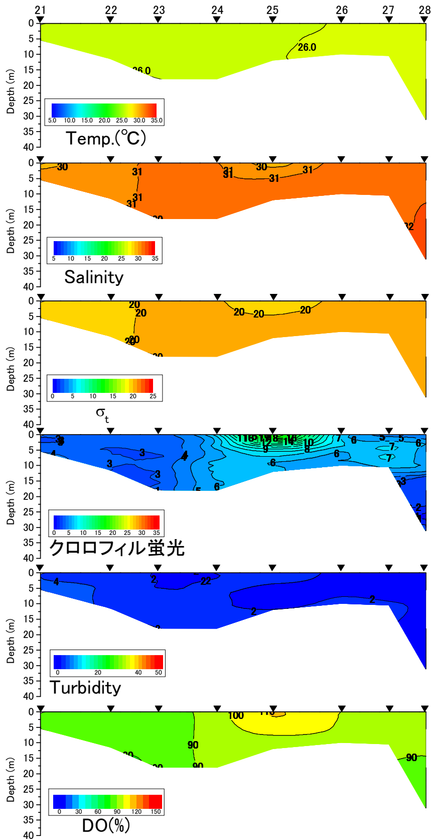
有明海東ラインの水温(°C)、塩分、密度( \sigma_t )、クロロフィル蛍光強度、濁度、溶存酸素飽和度(DO%)の鉛直面図(国土交通省の調査による) (2016年9月1日)
